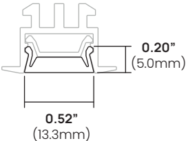
Louvers
